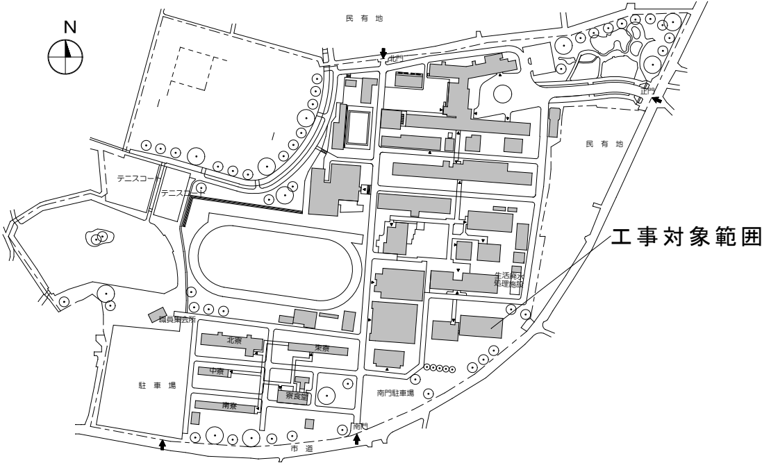
配置図
