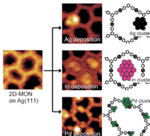
STM測定による、2次元多孔性有機金属薄膜へ金属を蒸着させて得られる金属クラスターのSTM像。
