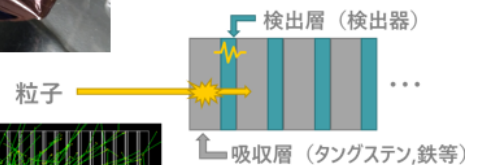
⇨ カロリメータの構造
