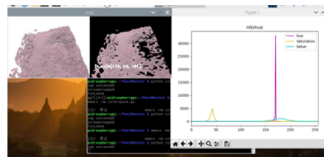
⇨ Webカメラを用いた材料の色相スペクトル評価
