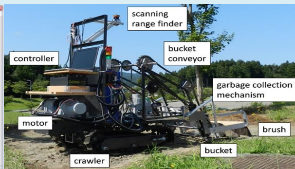
図4 海浜清掃ロボット
