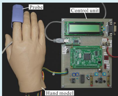
図3 蘇生訓練用生体シミュレータ
